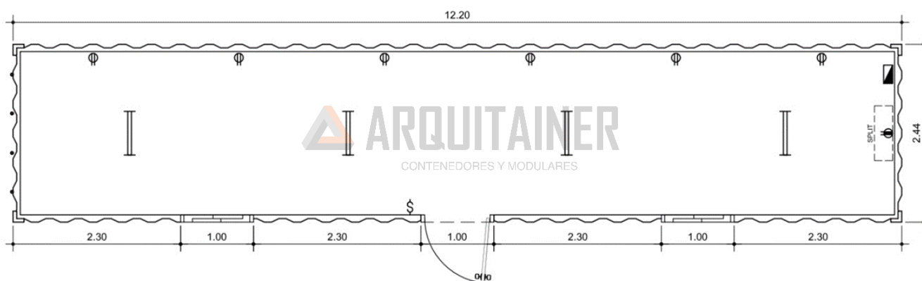
PLANTA DE CONTAINER 40' MODELO A _ OFICINA
